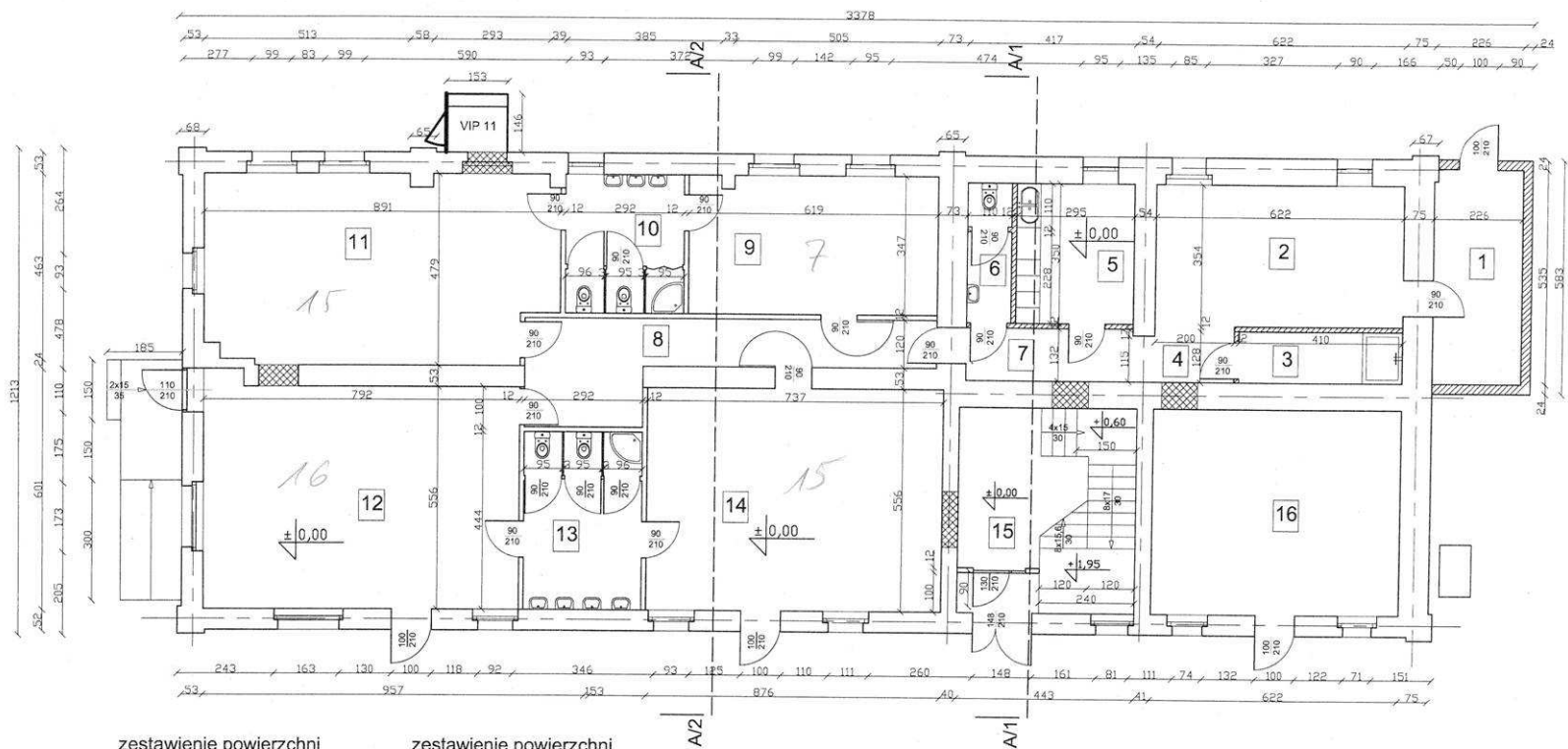
zestawienie powierzchni pomieszczeń przedszkola
